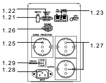
800VA~1500VA(220V)
