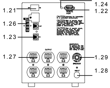
2200VA(110V)
