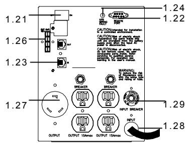
3000VA(110V)
