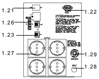
2200VA(220V)/3000VA(220V)
