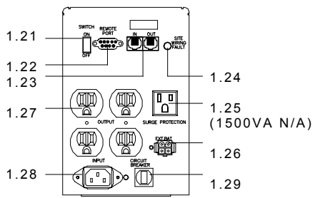
800VA~1500VA(110V)
